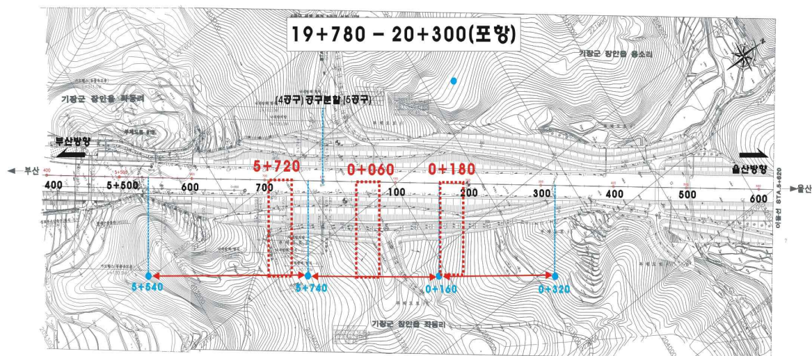
평면도
